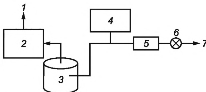
Рисунок 1 — Схема вакуумной системы для вакуумных капиллярных вискозиметров
