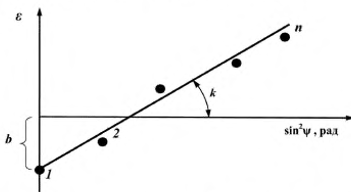
Рисунок 2 — Построение зависимости \varepsilon = k \sin^2 \psi + b для n наклонов нормали \psi к кристаллографической плоскости
