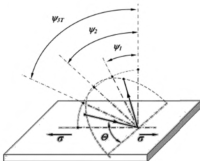
Рисунок 1 — Схема измерения для различных углов \psi
