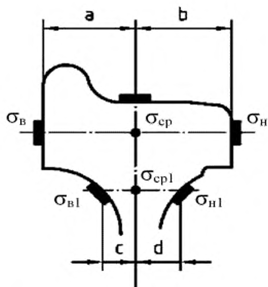
Рисунок А.6 — Схема приведения к плоскости круга катания ( \sigma_{ср} и \sigma_{ср1} ) напряжений, замеренных ( \sigma_в , \sigma_н , \sigma_{в1} , \sigma_{н1} ) на боковых поверхностях обода (бандажа) и прибородной части диска
