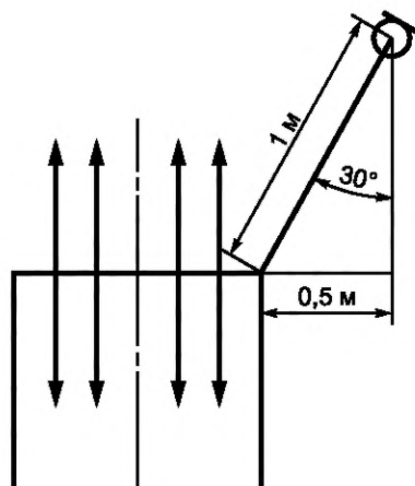
Рисунок 2 — Измерительные точки у всасывающего или выхлопного патрубка
