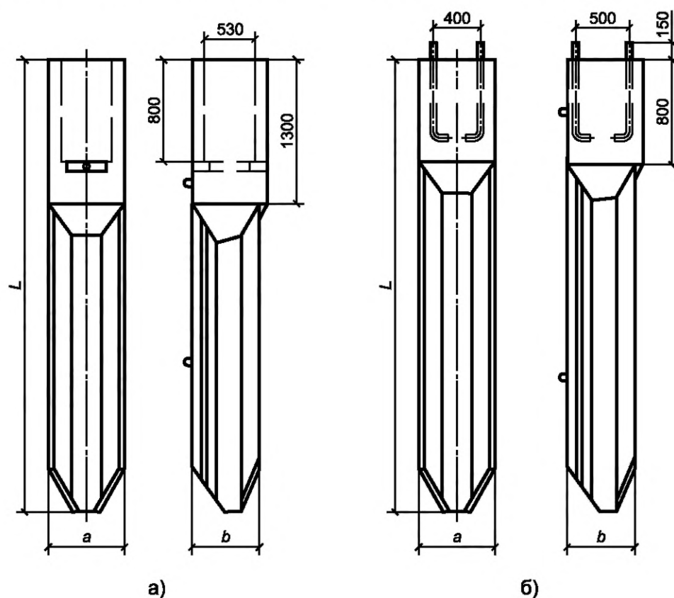
Рисунок 1 — Трехлучевые фундаменты: а) со стеканным креплением стоек; б) с анкерным креплением стоек
