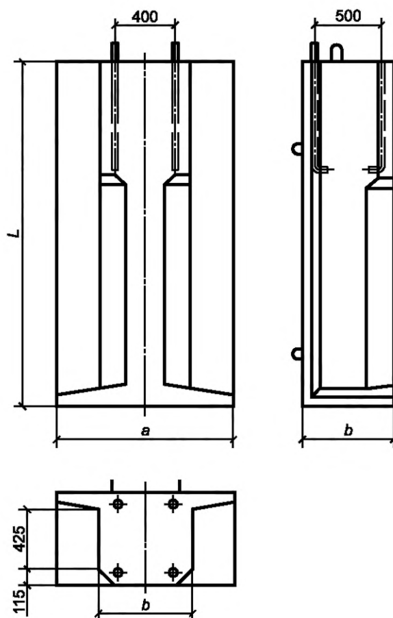
Рисунок 4 — Фундамент с уширенной полкой
