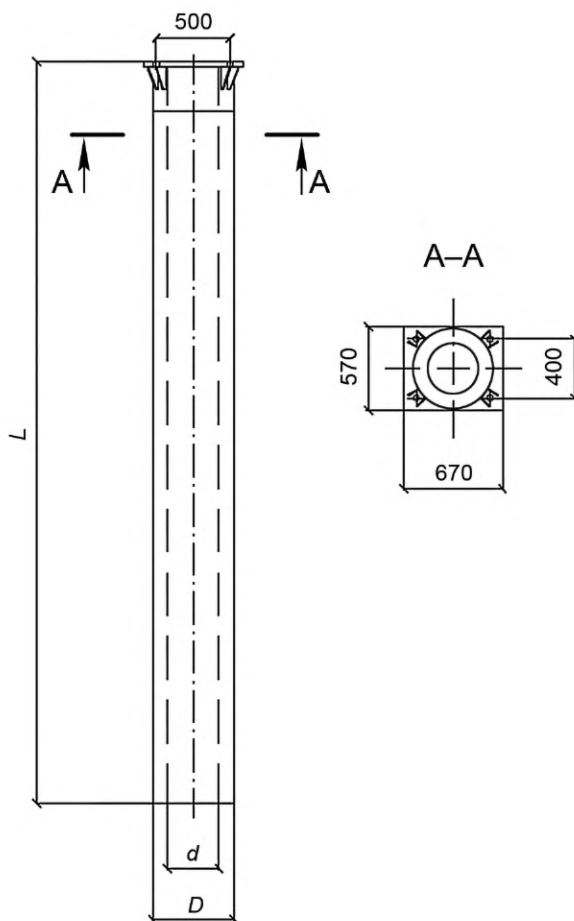
Рисунок 4б — Свая цилиндрическая фланцевая.
