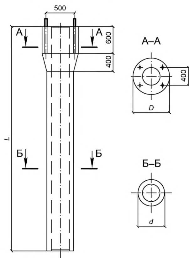
Рисунок 4а — Фундамент цилиндрический полый
