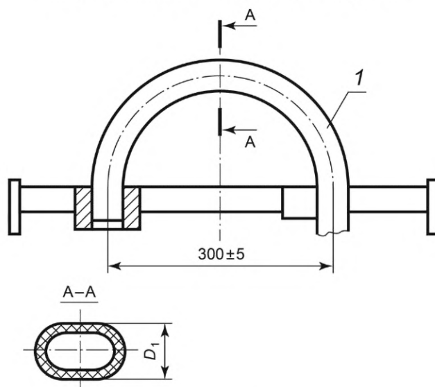
Схема приспособления для изгиба рукава
