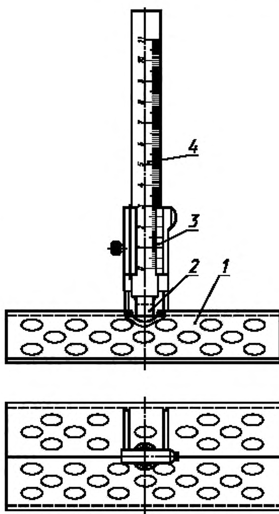
1 — основание; 2 — наконечник; 3 — конус; 4 — измерительный стержень
