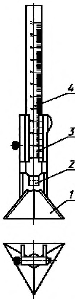
1 — основание; 2 — наконечник; 3 — конус; 4 — измерительный стержень
