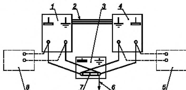
1 — первая стойка испытуемого ТС АС; 2 — линия связи между стойками; 3 — опорный узел заземления ТС АС; 4 — л-я стойка испытуемого ТС АС; 5 — подключение ИГ к л-й стойке испытуемого ТС АС; 6 — цепь связи с физической землей; 7 — перемычки между сигнальной и защитной системами заземления; 8 — подключение ИГ к первой стойке испытуемого ТС АС
