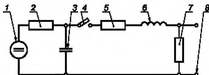
1 — источник высокого напряжения; 2 — зарядный резистор; 3 — зарядный конденсатор; 4 — коммутающий ключ; 5 — резистор цепи формирования длительности импульса, определяющий внутреннее сопротивление ИГ; 6 — индуктивность цепи формирования длительности фронта импульса; 7 — резистор цепи формирования длительности импульса; 8 — к испытуемой цепи ТС АС
