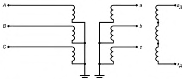
A, B, C — фазы первичной обмотки ТН; a, b, c — фазы основной вторичной обмотки ТН; a_d, x_d — фазы дополнительной вторичной обмотки ТН
