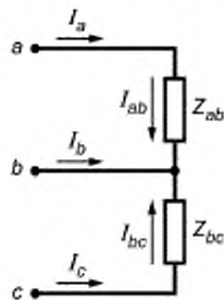
a, b, c — фазы основной вторичной обмотки ТН; I_a, I_b, I_c — фазные токи; I_{ab}, I_{bc} — междофазные токи; Z_{ab}, Z_{bc} — междофазные нагрузки
