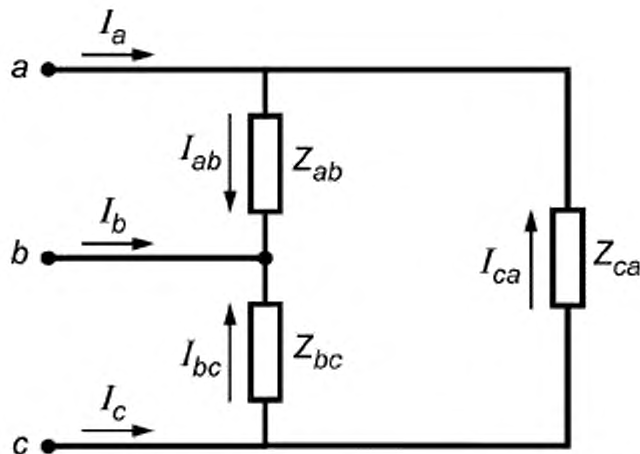
Рисунок Б.6 — Схема соединения нагрузок ТН треугольником для трехпроводной вторичной цепи
