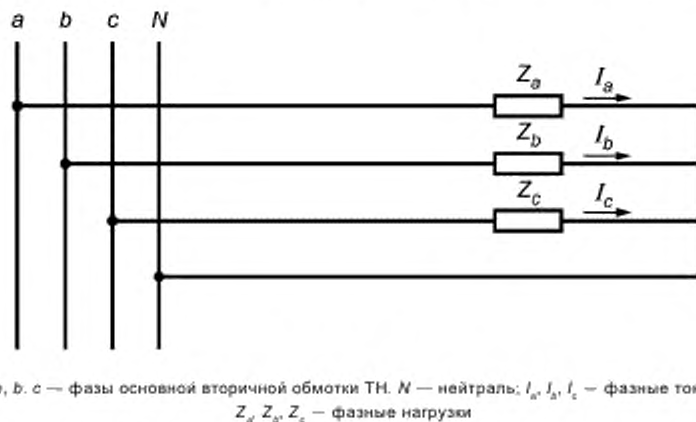
Рисунок Б.7 — Схема соединения нагрузок ТН для четырехпроводной измерительной цепи
