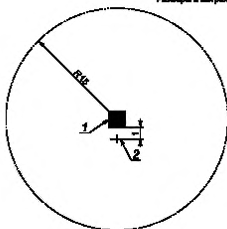
1 — испытуемый образец на пластине заземления, 2 — антенна
