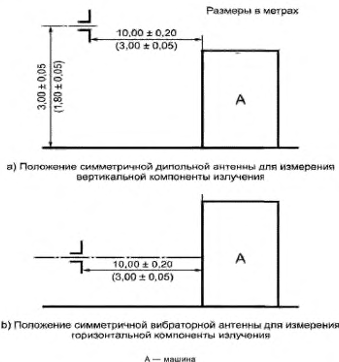
Рисунок В.2 — Расположение антенны относительно машины при измерениях
