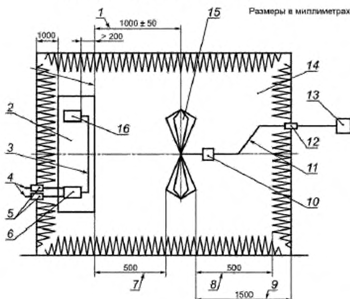
Рисунок D.1 — Открытая измерительная площадка
