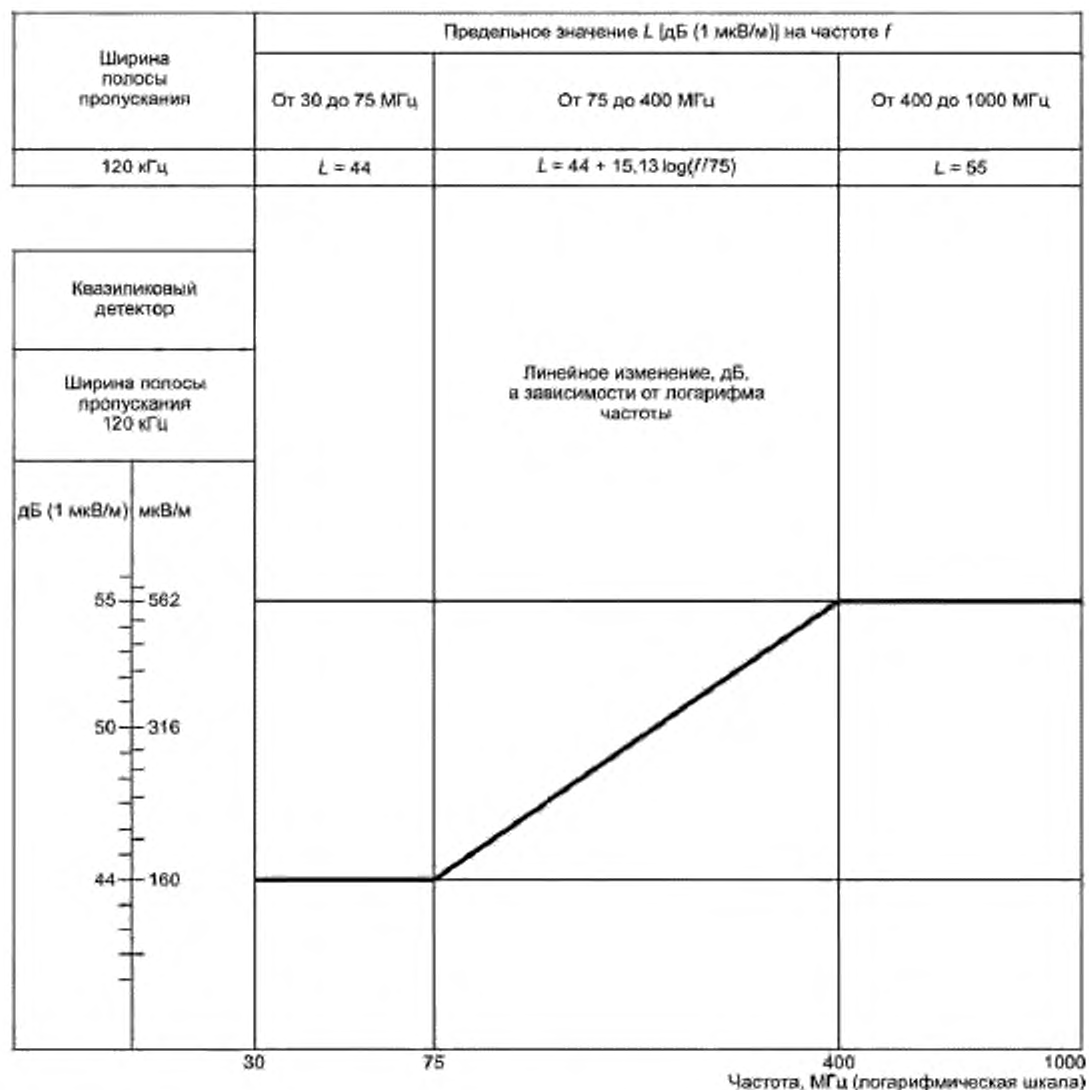
Рисунок А.2 — Контрольные предельные уровни широкополосных электромагнитных помех, создаваемых машинами (расстояние от машины до антенны 3 м)
