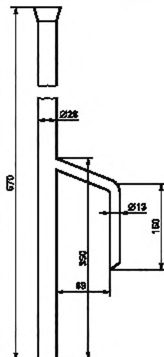
Рисунок А.1 — Пробирка с отводом
