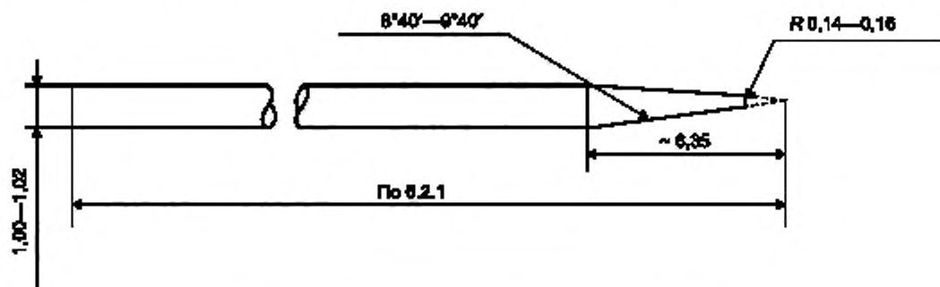
Рисунок 1 — Игла для определения пенетрации
