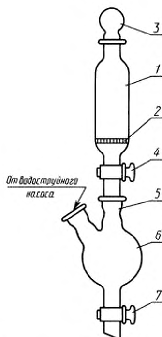
Экстрактор
