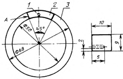
1—отверстие для термопары; 2—образец (колодка); 3—заготовка
