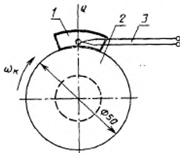
1 — образец (колодка); 2 — контртело (диск); 3 — термопара
