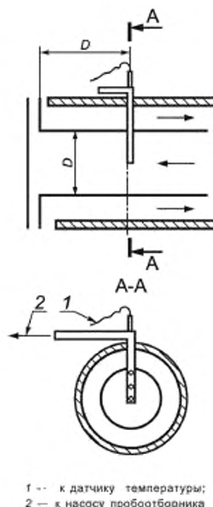
Рисунок 12 — Пробоотборник для водонагревателей типа С
