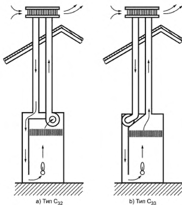
Рисунок В.3 — Водонагреватели типа C 3
