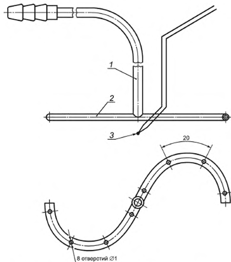
Рисунок 10 — Пробоотборник для отбора проб продуктов сгорания для испытательных дымоходов диаметром D < 100 мм
