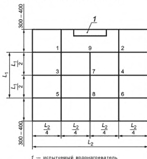
1 — испытуемый водонагреватель
