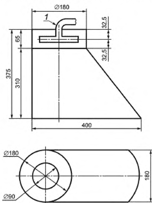
Т — пробоотборник (рисунок 7)
