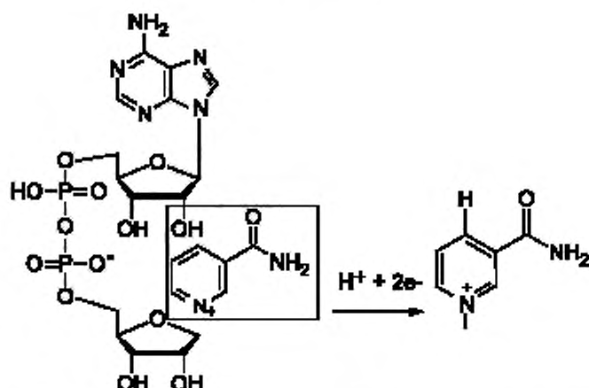
Рисунок Б.2 — Реакция обратимого окисления никотинамидадениндинуклеотида
