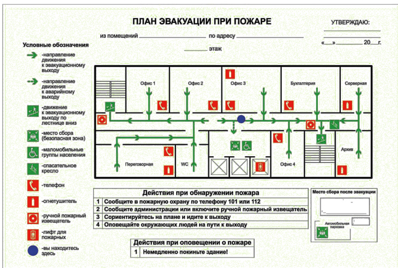
Рисунок 9 — Пример плана эвакуации
