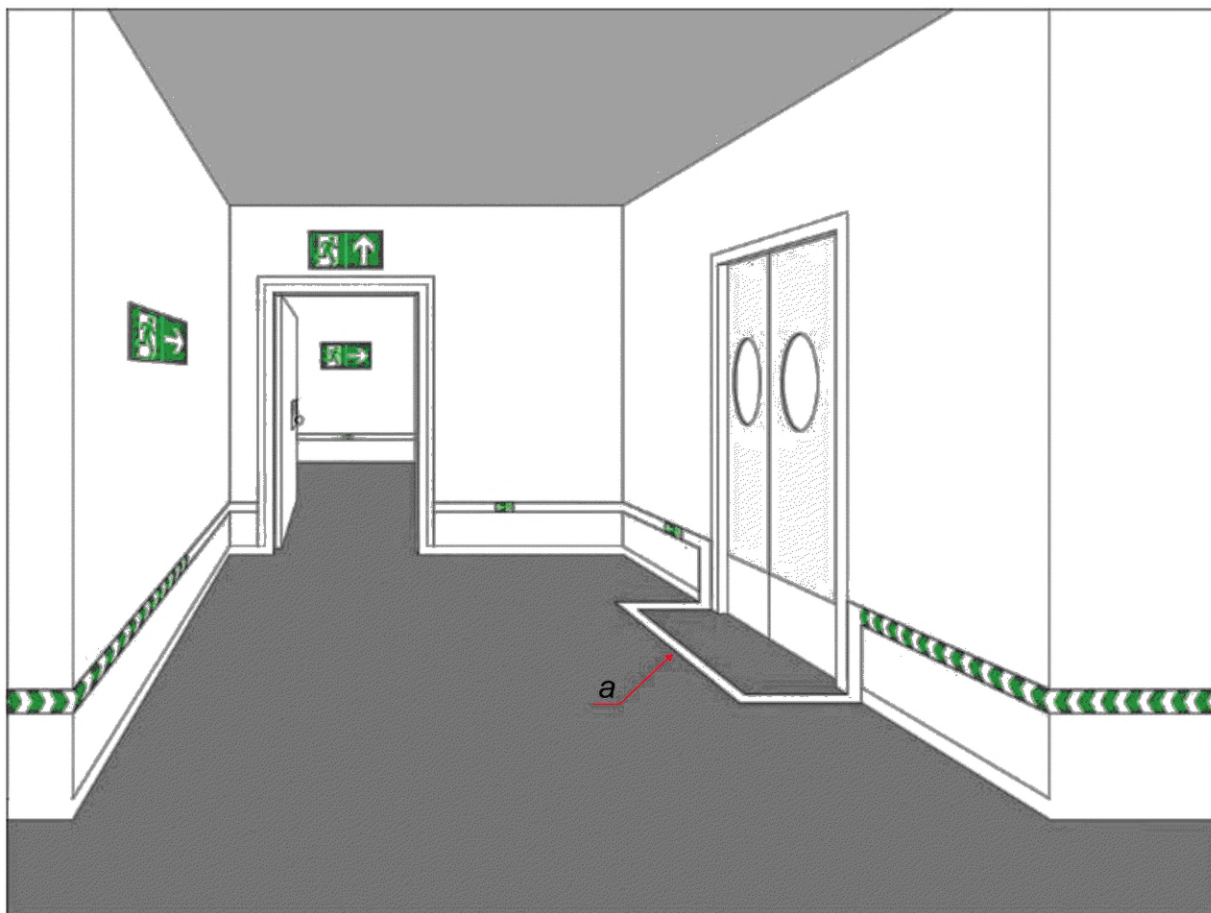
Рисунок В.10 — Пример обозначения дверей шириной более 1 м вдоль путей эвакуации в коридорах, проходных помещениях и т. п.
