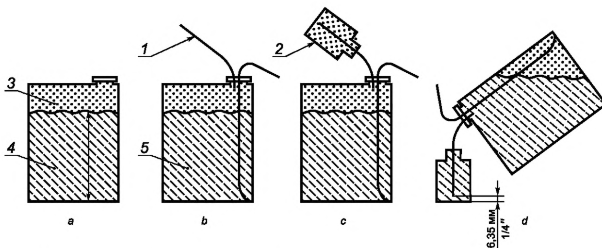
1 — трубка для переноса охлажденной пробы; 2 — охлажденная жидкостная камера; 3 — пар; 4 — жидкость; 5 — охлажденный образец a — контейнер с пробой для переноса пробы; b — герметичный затвор заменен соединением для переноса пробы; c — бензиновая камера, помещенная над трубкой подачи жидкости; d — положение системы при переносе пробы
