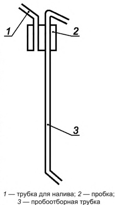
Рисунок А1.2 — Приспособление для переноса пробы
