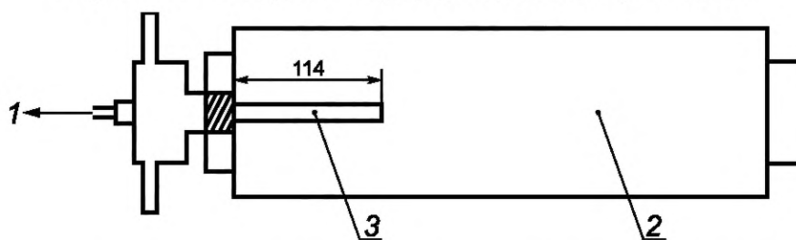
Рисунок A2.1 — Аппарат для определения давления паров. Метод В
