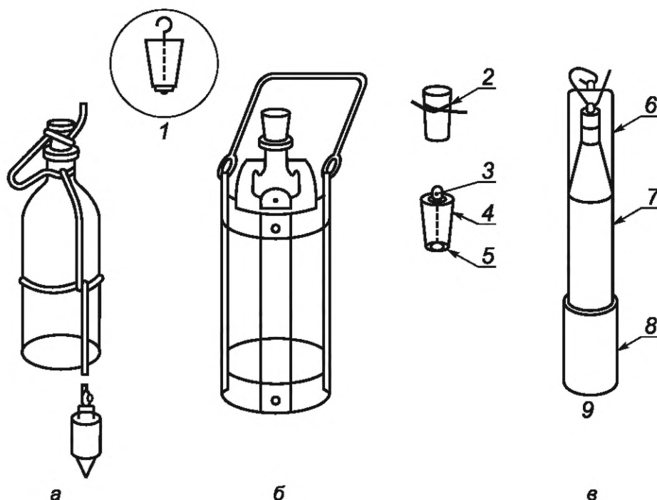
а — собранный пробоотборник; б — обрешетка (держатель, клеть) для утяжеления пробоотборной бутылки вместимостью 1 л (1 кварта) (изготовлена для бутылки любого размера); в — утяжеленный пробоотборный стакан вместимостью 1 л (1 кварта); 1 — деталь пробки; 2 — крепежное устройство; 3 — ушко пробки; 4 — пробка; 5 — прокладка пробки; 6 — держатель из медной проволоки; 7 — ушки из медной проволоки; 8 — свинцовый чехол; 9 — стакан
