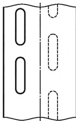
Рисунок 2 — Напорная труба (с перекрывающимися отверстиями)
