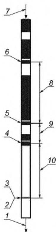
1 — нижняя часть; 2 — фронт элюирования; 3 — чистая жидкость; 4 — первая интенсивная желтая флуоресценция; 5 — первая интенсивная голубая флуоресценция; 6 — красное кольцо; 7 — верхняя часть; 8 — зона ароматических углеводородов; 9 — зона олефинов; 10 — зона насыщенных углеводородов
