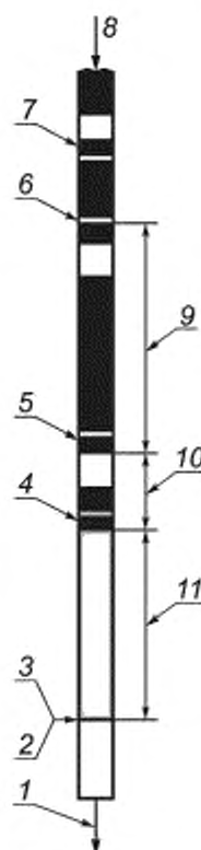
1 — нижняя часть; 2 — фронт элюирования; 3 — чистая жидкость; 4 — первая интенсивная желтая флуоресценция; 5 — первая интенсивная голубая флуоресценция; 6 — красно-коричневое кольцо; 7 — дополнительное красное кольцо; 8 — верхняя часть; 9 — зона ароматики; 10 — зона олефинов; 11 — зона насыщенных углеводородов
