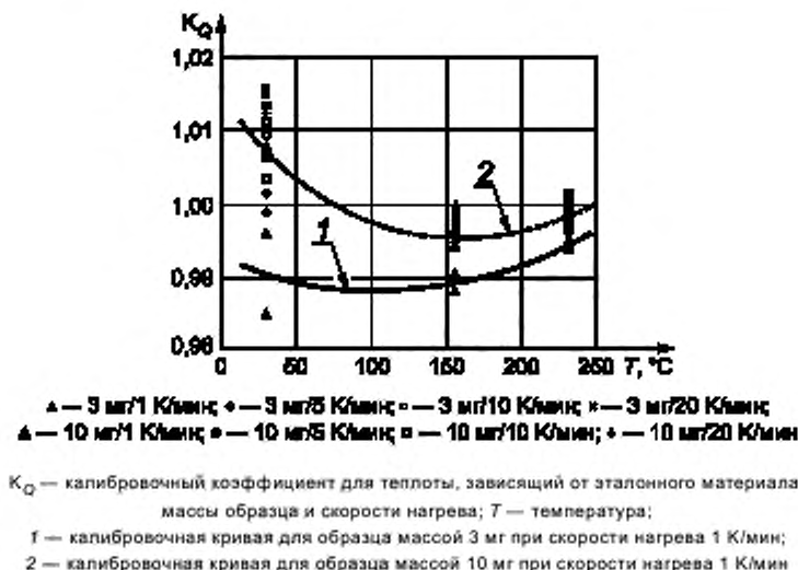
Рисунок ДА.7 — Калибровочные кривые по теплоте, полученные с использованием галлия, индия и олова
