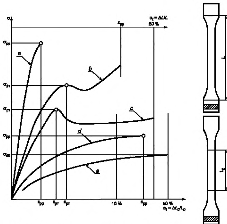
Рисунок 1 — Определение предела текучести при растяжении \sigma_{рп} относительного удлинения при пределе текучести \epsilon_{рп} , разрушающего напряжения при растяжении \sigma_{рр} , относительного удлинения при разрыве \epsilon_{рр} , номинального относительного удлинения при разрыве \epsilon_{ррн} и растягивающего напряжения при 50%-ном относительном удлинении \sigma_{50} по кривым «напряжения — деформации»
