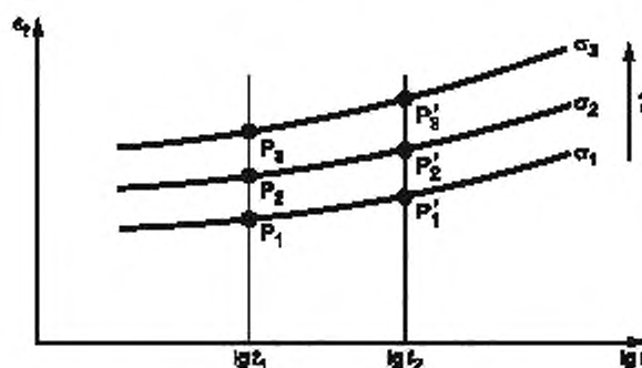
Рисунок 2 — Кривые ползучести
