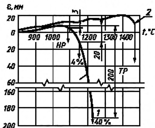
Диаграмма «Температура — деформация»
