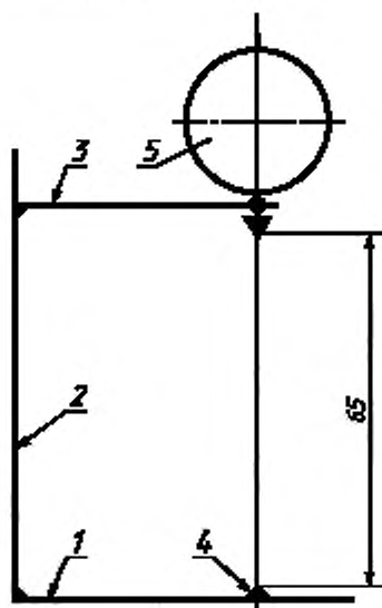
Схема штатива с индикатором часового типа
