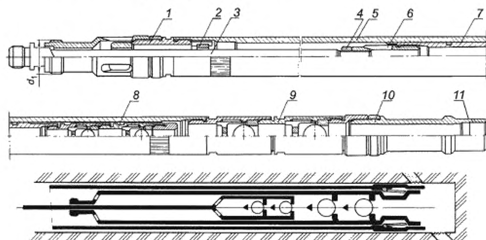
1 — защитный клапан; 2 — упор; 3 — шток; 4 — контргайка; 5 — цилиндр; 6 — переводник плунжера; 7 — плунжер; 8 — замковая опора; 9 — всасывающий клапан; 10 — упорный nipple с конусом; 11 — переводник насоса
