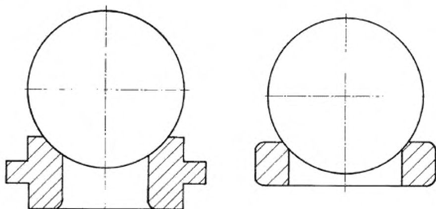
а — клапан КБ; б — клапан К
