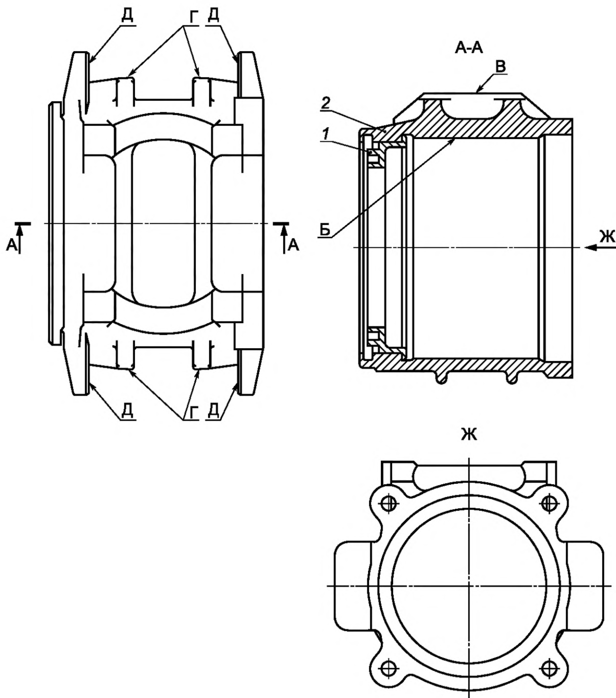
1 — лабиринтная часть; 2 — корпус буксы; Б — опорная поверхность под подшипник; В — опорная поверхность под боковую раму; Г — упорные стенки ограничителей продольных перемещений; Д — ограничители боковых перемещений; Ж — вид сбоку
