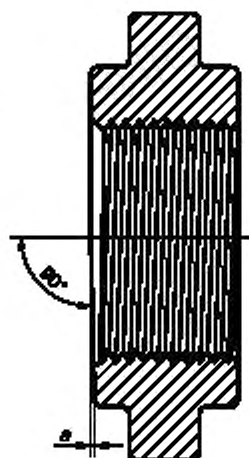
Рисунок 17 — Контргайка для удлинения крейцкопфа и штока поршня
