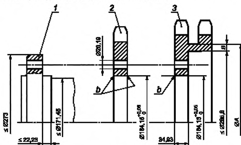
Рисунок 10 — Съемные цепные звездочки
