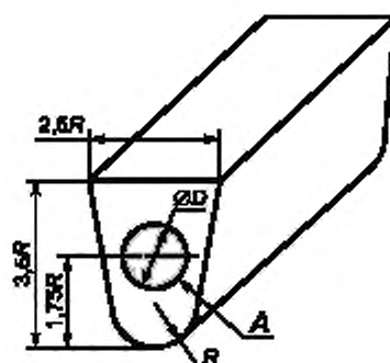
Рисунок 3 — Эквивалентные круговые модели. Деталь с конфигурацией кильблока
