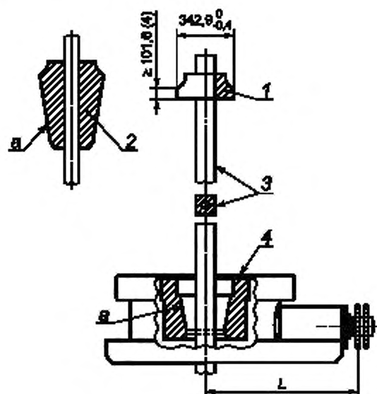
1 — втулка с квадратным хвостовиком, извлеченная из ротора; 2 — клиновой захват для труб; 3 — ведущая буровая труба; 4 — постоянная втулка в разрезе; а — конусность 1:3 ( 330 \pm 1,5 ) мм/м
