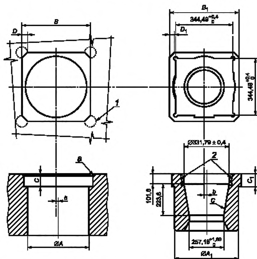
1 — вариант конфигурации. 2 — стандартная конфигурация; а — фаска \geq 6 мм 45^\circ ; b — эксцентриситет \leq 0,40 мм; c — конусность 1:3 ( 330 \pm 1,5 ) мм/м
