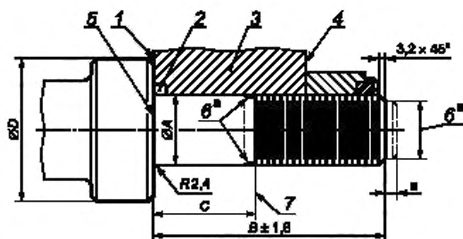
1 — заплечик N, заплечик плунжера, торец штока; 2 — необходимое уплотнение, размеры выбираются по усмотрению производителя; 3 — плунжер; 4 — заплечик P, заплечик плунжера, конец резьбы; 5 — заплечик M, заплечик штока; 6 — спад затылка на резьбе, конфигурация по усмотрению производителя; 7 — калибровочная часть резьбы, а — дополнительная возможность удлинения
