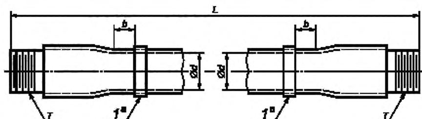
T — предохранительный хомут, L — номинальная длина, b — место для пометки «Место для установки присоединительного хомута»; b — для бурового шланга данная величина составляет от 150 до 460 мм от внутреннего края соединения; для шлангов вибратора размер составляет от 150 до 250 мм от внутреннего края соединения
