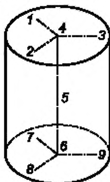
Рисунок Б.1 — Положение термодатчиков (1—9) в цилиндрических печах
