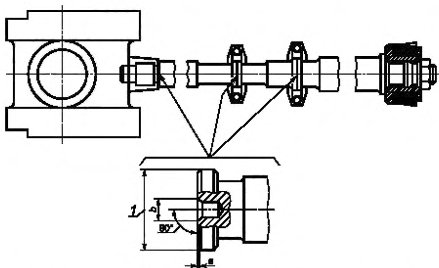
f — диаметр торца, a — плоские поверхности контакта и посадочные диаметры на сопряженных соединениях удлинения ползуна со ступицей поршня в буровых насосах; b — допуск соосности между осевой линией посадочного диаметра и теоретической осью штока не должен превышать 0,13 мм
