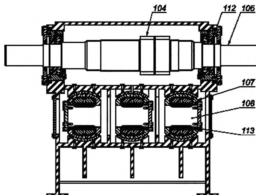
Рисунок В.3 — Поперечное сечение через вал-шестерню и крейцкопф (номенклатура деталей см. в таблице В.1)
