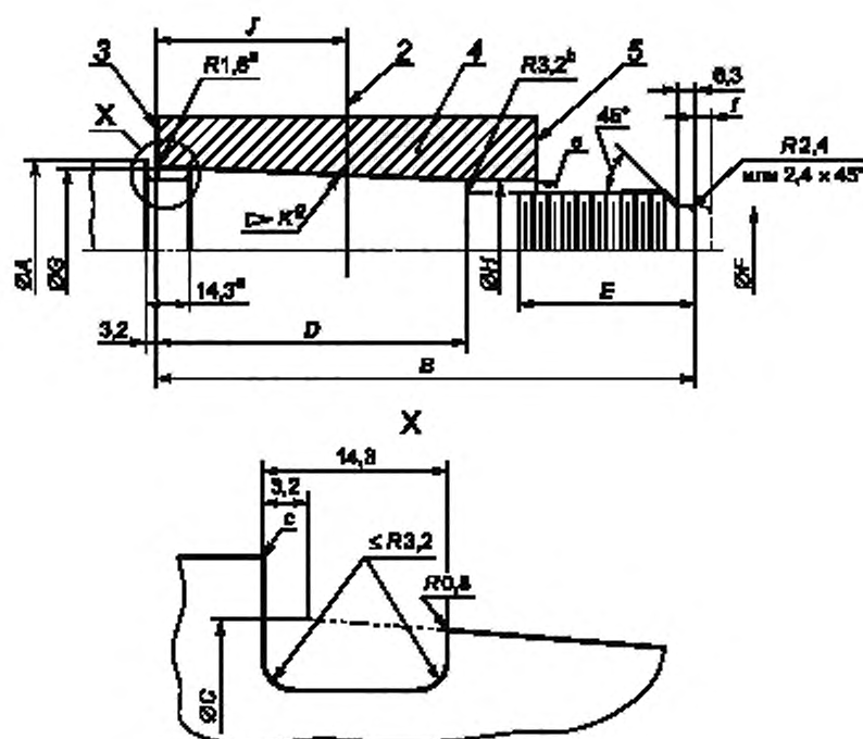
1 — заплечик штока М; 2 — геометрическая ось поршня (в сборе); 3 — заплечик N, заплечик поршня, штоковая полость; а — максимальный размер; б — минимальный размер; в — фаска \leq 0,5 мм; J — длина до центральной оси поршня; B — длина штоковой полости; X — галтель и диаметр выточки, накатанной при холодной обработке; 4 — поршень; 5 — заплечик P, заплечик поршня, конец резьбы; 6 — фаска; f — максимальное удлинение хвостовика 3,2 мм; g — конус; R — радиус или фаска
