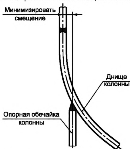
Рисунок 5 — Узел стыковки опорной обечайки и днища аппарата
