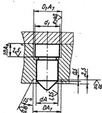
Пример применения рассекателя в сменной пресс-форме
