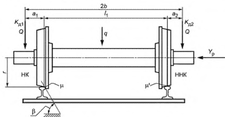
Рисунок 2 — Расчетная схема для формул (81) и (82)
