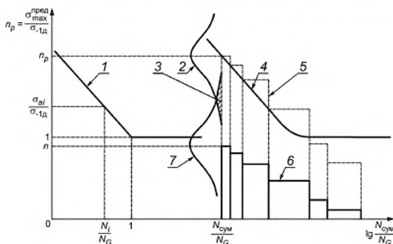
1 — первичная кривая усталости; 2 — закон рассеяния кривой усталости; 3 — зона амплитуд, вызывающих относительное повреждение детали; 4 — вторичная кривая усталости, соответствующая действующему блоку нагружения; 5 — предельный блок нагружения, пропорциональный действующему блоку, соответствующий заданному числу циклов N_{сум} ; 6 — действующий блок нагружения; 7 — закон рассеяния действующего блока нагружения.
