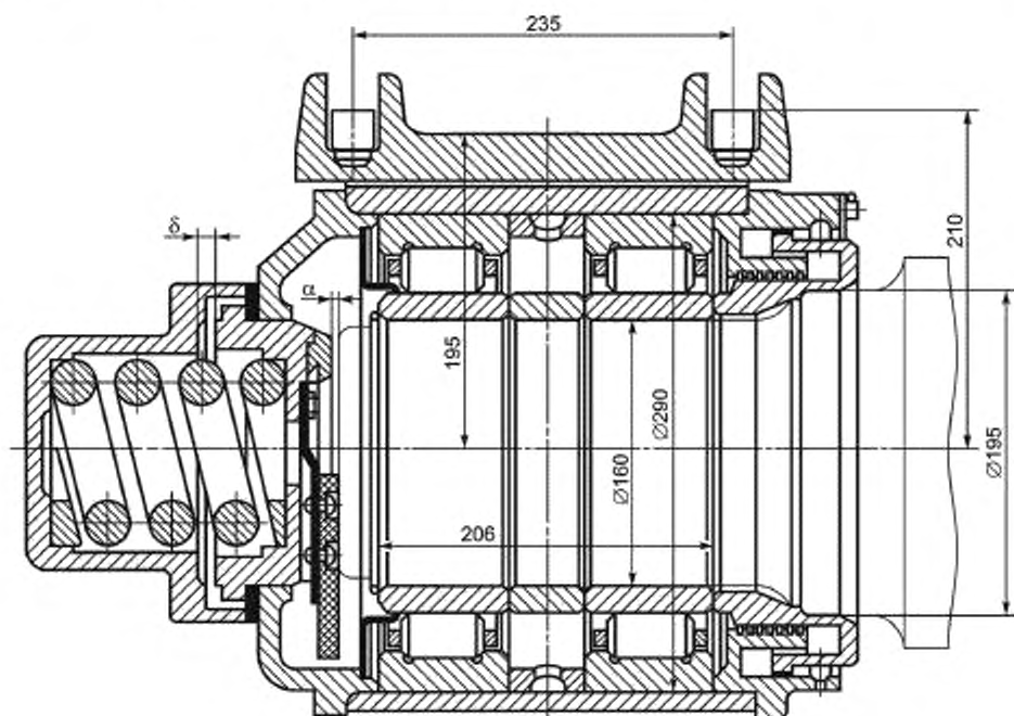
Рисунок Г.1 — Букса колесной пары тепловоза ТЭЗ
