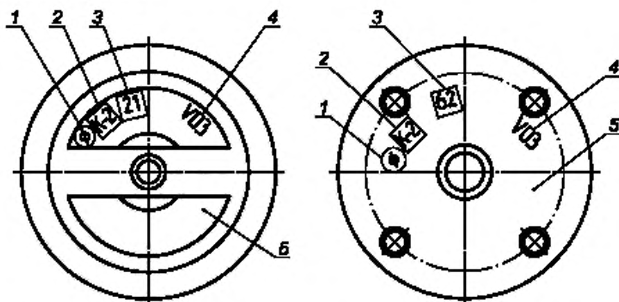
а) под подшипники качения с креплением гайкой
