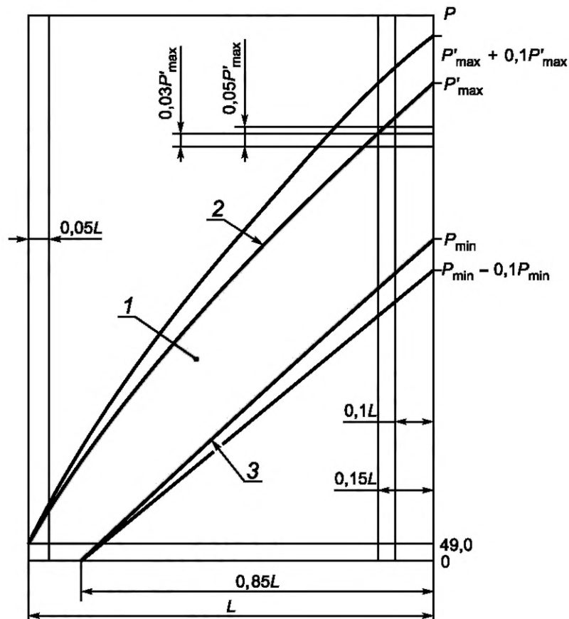
Рисунок 3 — Шаблон-диаграмма запрессовки
