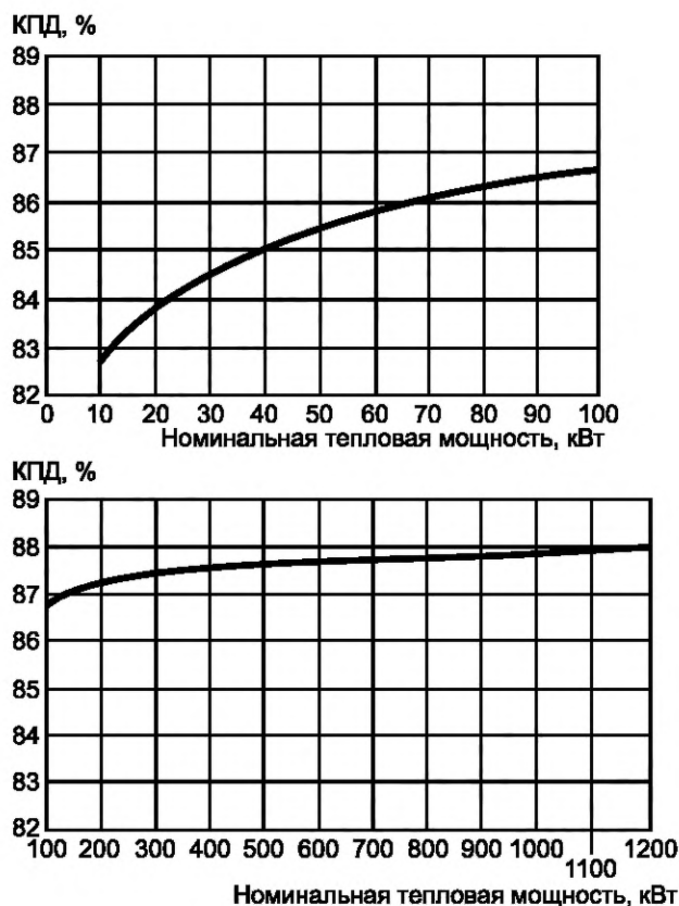
Рисунок 1 — График зависимости КПД рекуперативных воздухонагревателей от номинальной тепловой мощности
