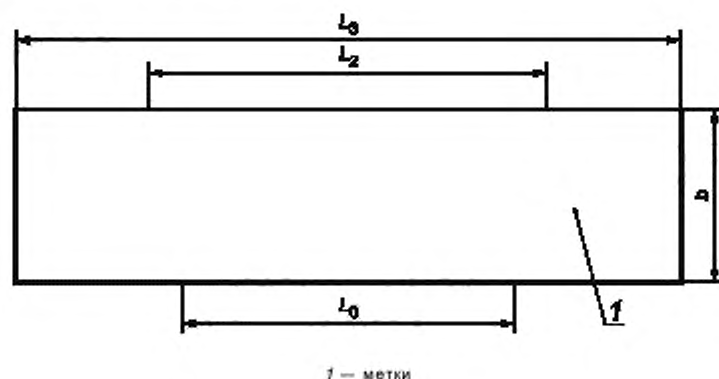
Рисунок 1 — Образец-полоска (метод А)
