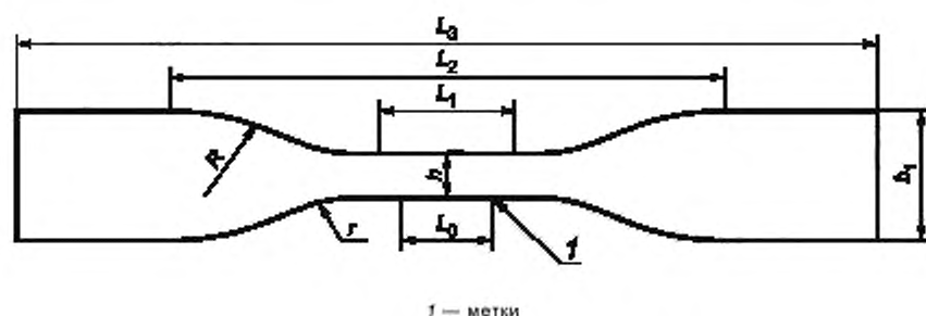
Рисунок 2 — Образец-лопатка (метод В)
