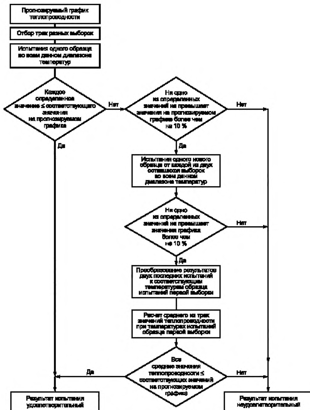
Рисунок 1 — Схема подтверждения теплопроводности
