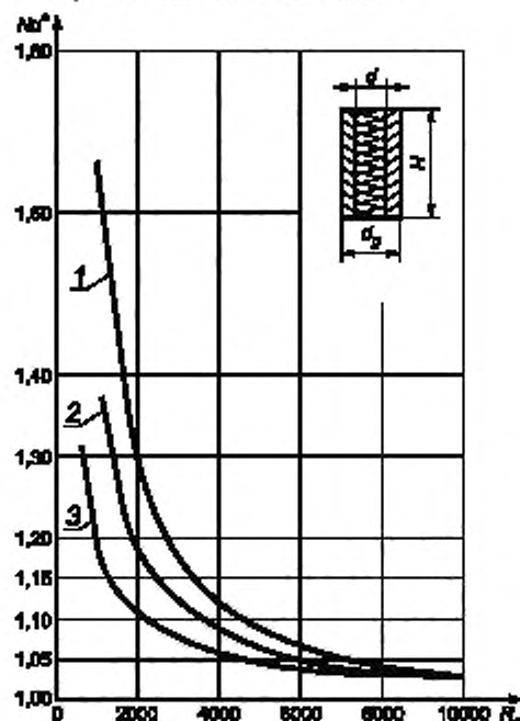
Рисунок А.4 — Диаграмма для теплоизоляционной системы общей толщиной d_g = 0,20 м
