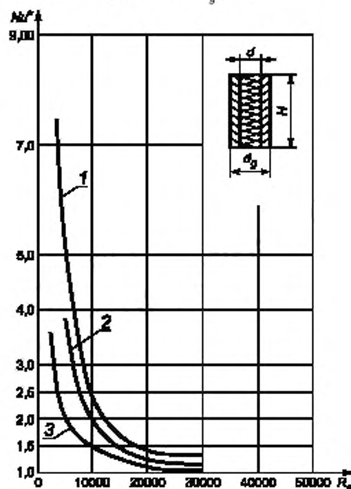
Рисунок А.6 — Диаграмма для теплоизоляционной системы общей толщиной d_g = 0,60 \text{ м}
