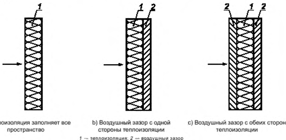
Рисунок А.3 — Виды систем теплоизоляции
