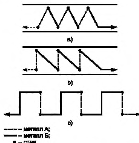
Рисунок Д.7 — Примеры расположения спаев термопар термобатареи
