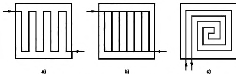
Рисунок D.6 — Схемы конструктивных решений трубок холодильника
