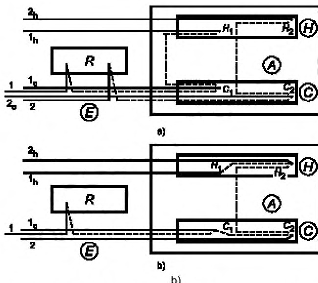
Рисунок D.5 — Соединения термодпар
