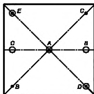
Рисунок D.4 — Расположение термодатчиков на рабочих поверхностях плит нагревателя и холодильника
