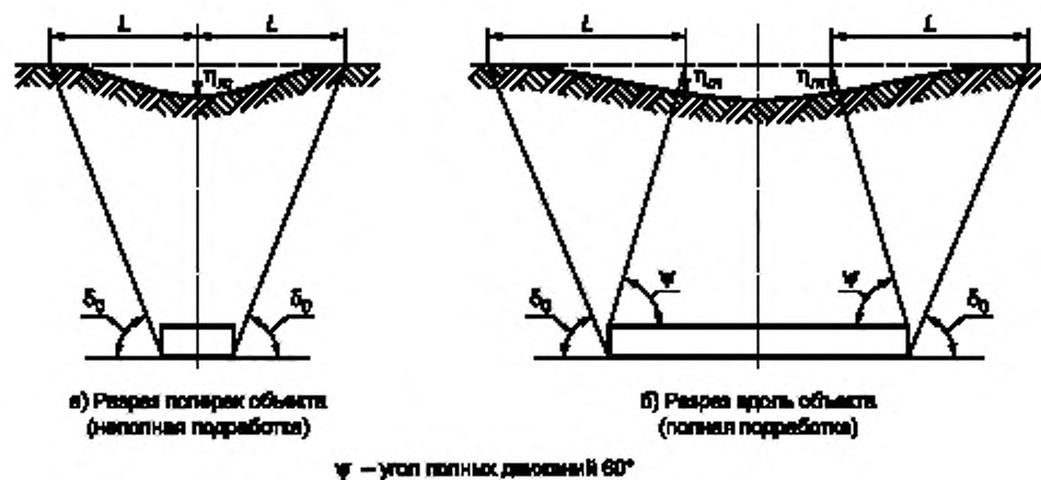
Рисунок Р.1 — Основные параметры мульты сдвижения
