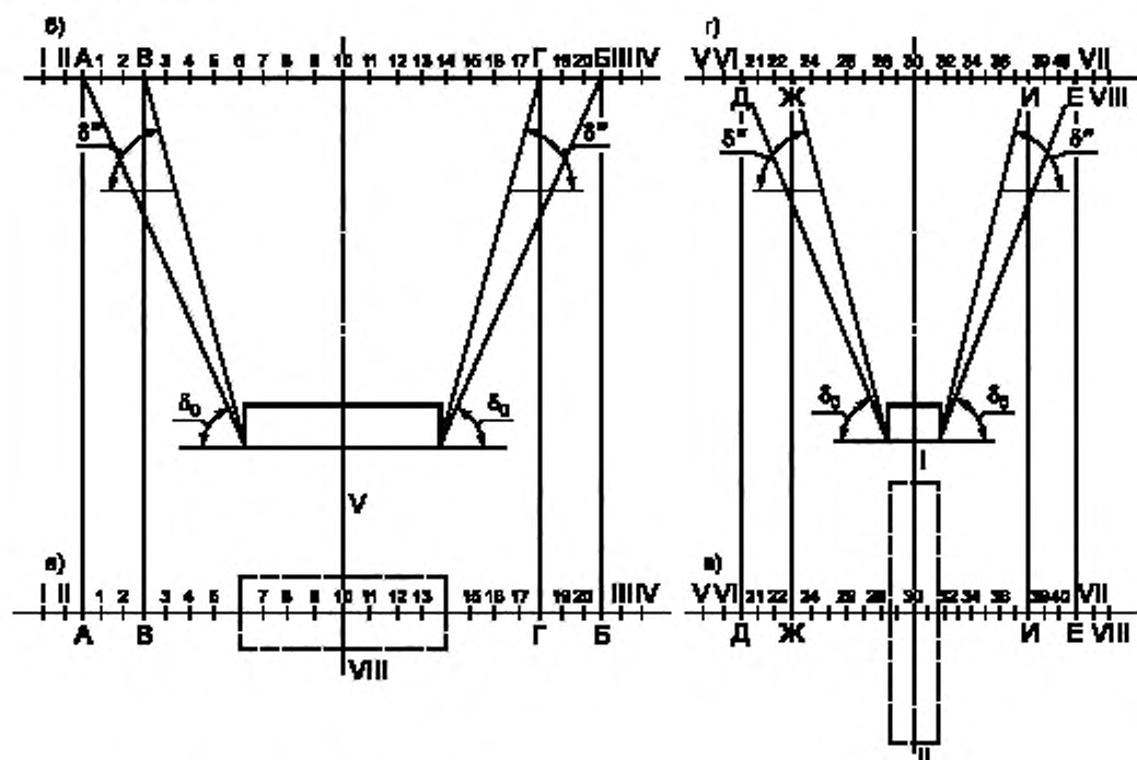
а) и б) — на плане и разрезе вдоль сооружения; в) и г) — на плане и разрезе поперек сооружения, I, II, III, IV, V, VI, VII, VIII — опорные реперы; 1—40 — рабочие реперы; АБ и ДЕ — зоны влияния подземного сооружения на земную поверхность; ВГ и ЖИ — зоны возможного образования трещин
