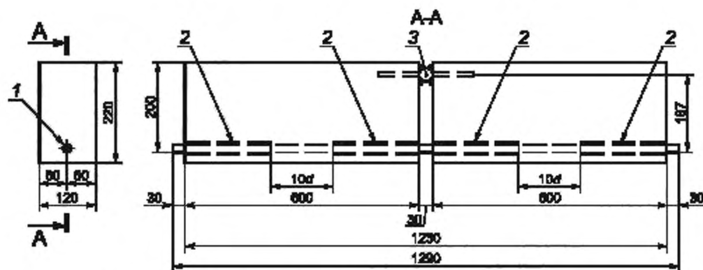
1 — стержень, 2 — поливинилхлоридный вкладыш или трубка; 3 — стальной цилиндр
