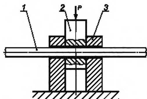
1 — испытательный образец; 2 — верхний нож; 3 — нижние ножи
