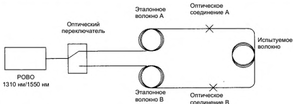
Рисунок D.1 – Расположение оптического переключателя
