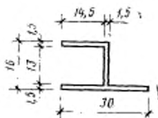
Профиль ПС 885—266
