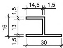
Рисунок В.1 — Профиль ПС 885-265
