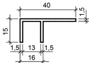
Рисунок В.1 — Профиль ПС 885-265
