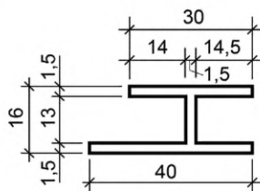
Рисунок В.2 — Профиль ПС 885-266
