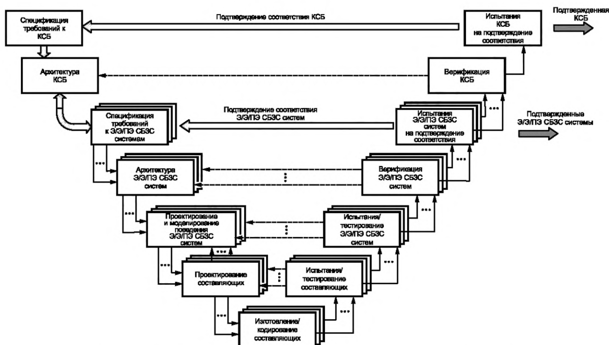
Рисунок 5 — V-образная модель стадий разработки и реализации ЖЦ КСБ
