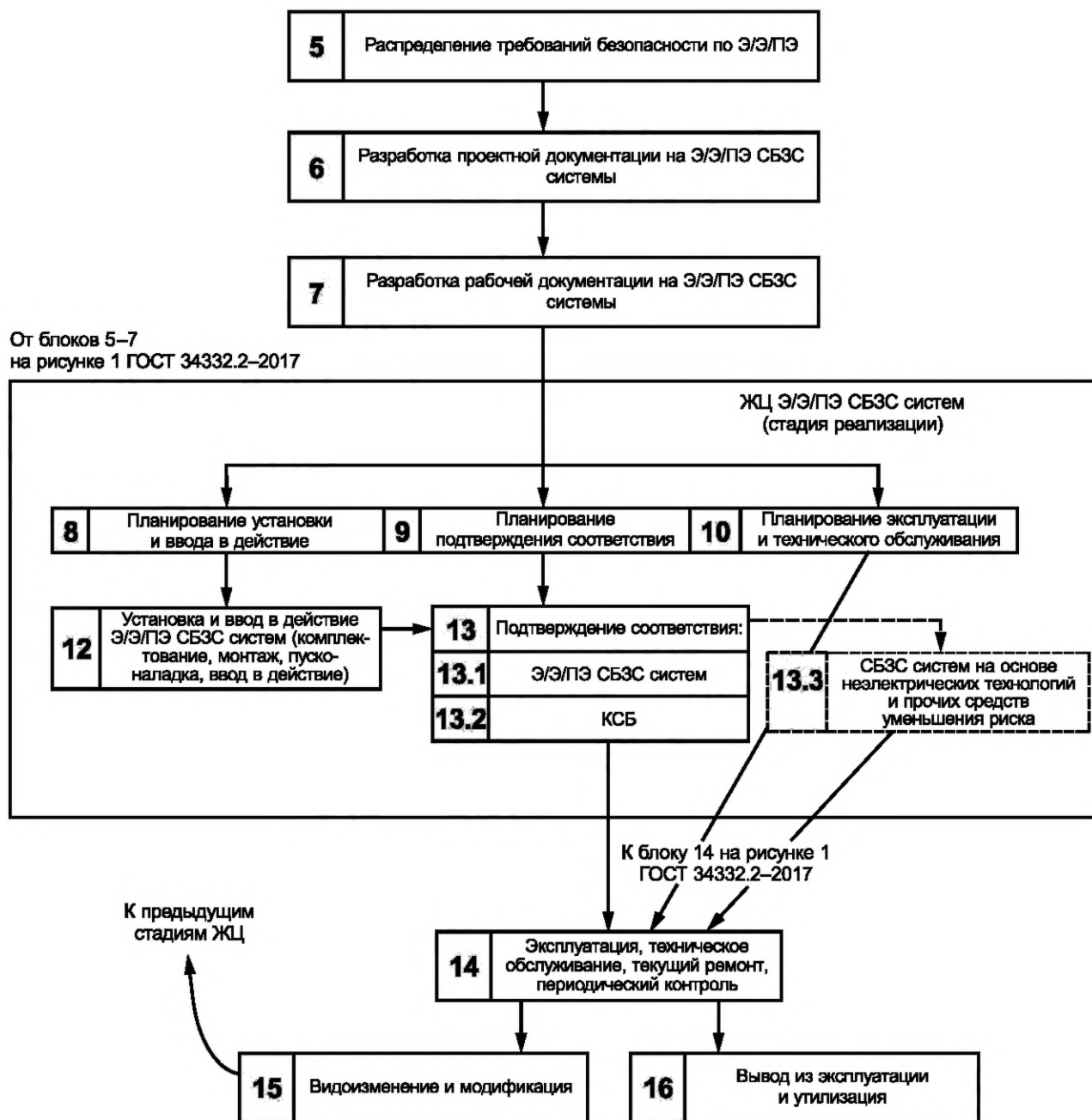
Рисунок 4 — Часть ЖЦ ПО ПЭ СБЗС системы
