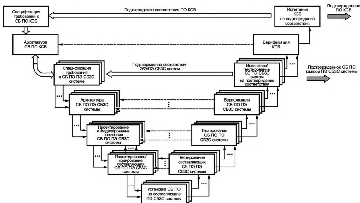
Рисунок 6 — V-образная модель стадий разработки и реализации ЖЦ СБ ПО КСБ
