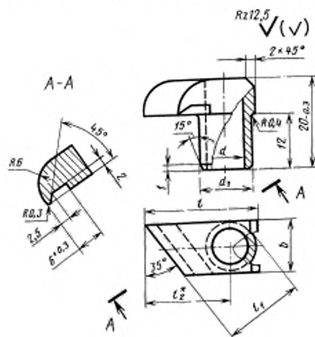
Прихват к резцам типов 1 и 2 (поз. 4)
