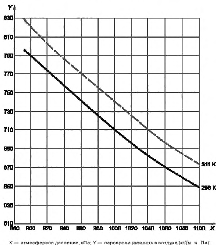
Рисунок В.1 — Зависимость паропроницаемости в воздухе от атмосферного давления в соответствии с формулой (В.4) при температурах 23 °С (296 К) и 38 °С (311 К)
