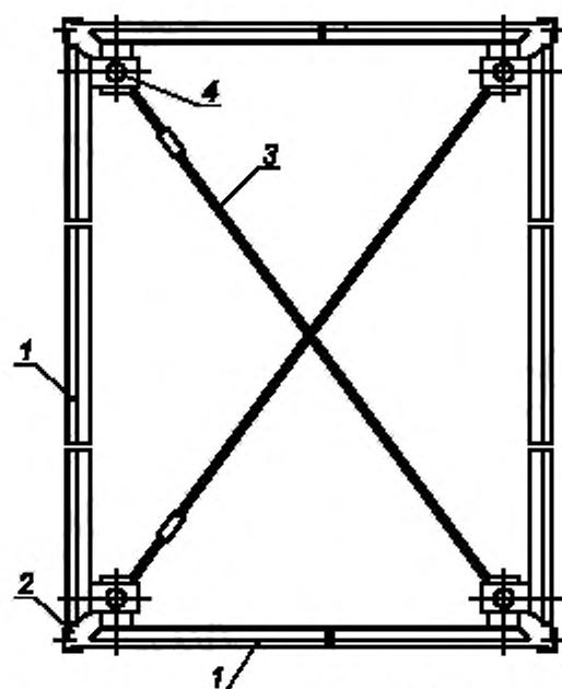
1 — щиты; 2 — угловые соединения; 3 — связи; 4 — вертикальная стойка
