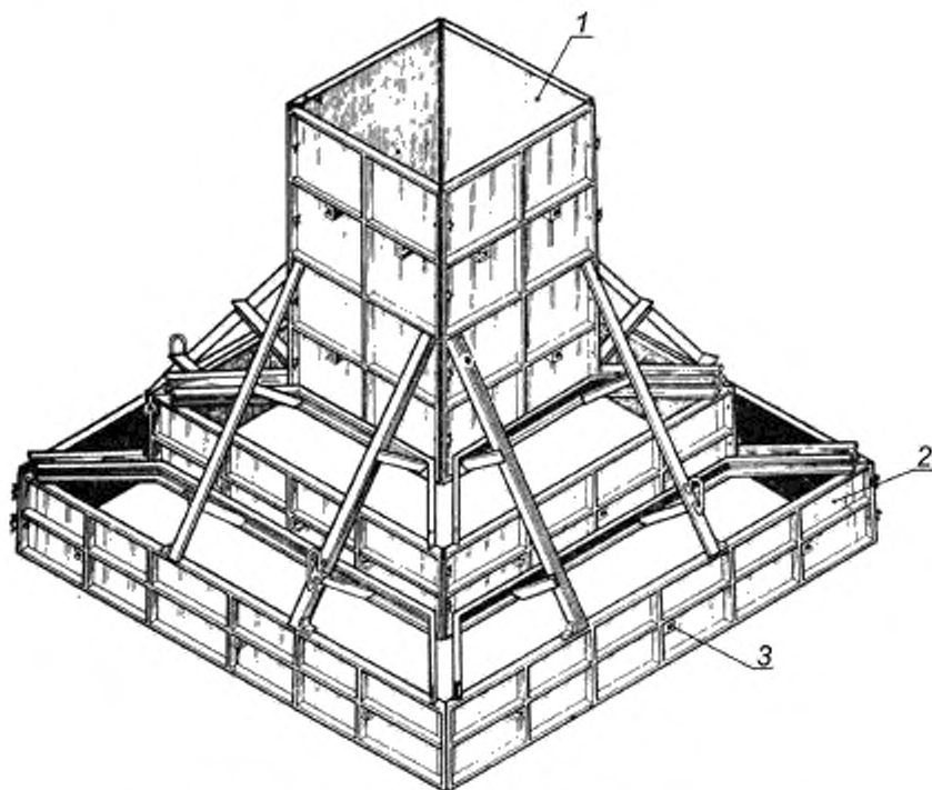
1 — опалубка подколонника; 2 — опалубка ступеней; 3 — отжимное устройство
