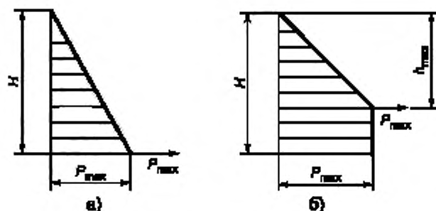
а — гидростатическое давление; б — расчетное давление при уплотнении смеси внутренними вибраторами
