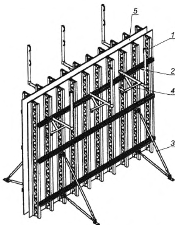
1 — вертикальные фермы; 2 — схватки; 3 — подкос; 4 — подмости; 5 — палуба (фанера)
