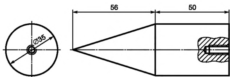
Рисунок 1 — Испытательный конус
