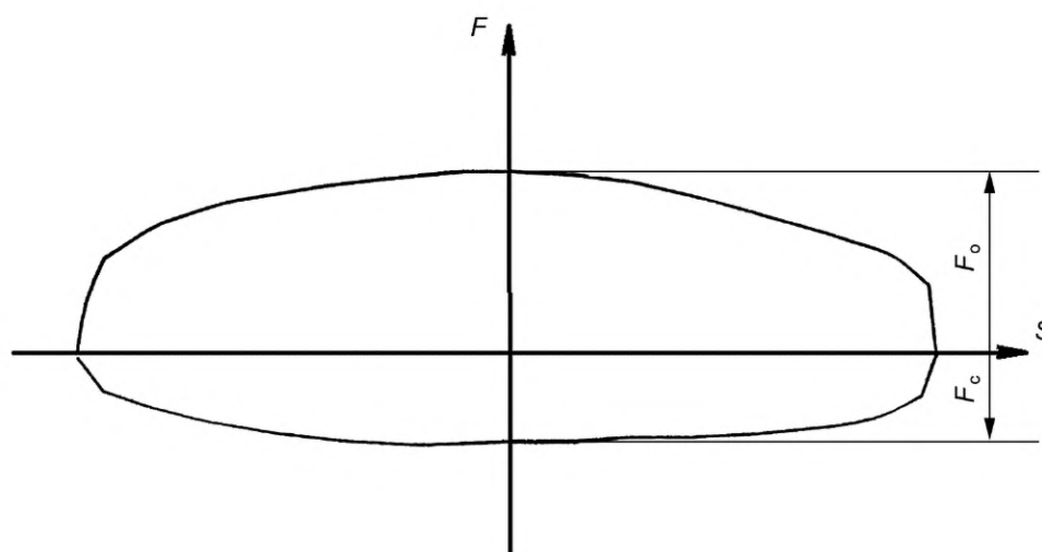
Рисунок 2 — Рабочая диаграмма при работе амортизатора с открывающимися клапанами отбоя и сжатия
