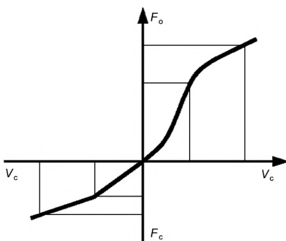
Рисунок 4 — Зависимость сопротивления амортизатора от скорости перемещения поршня
