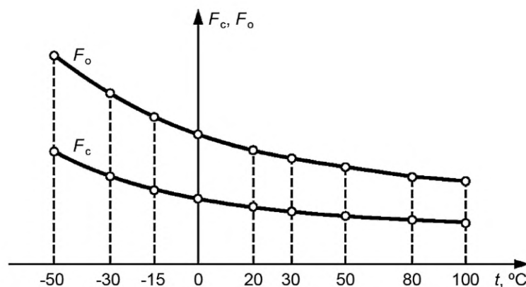
Рисунок 5 — Температурная характеристика амортизатора
