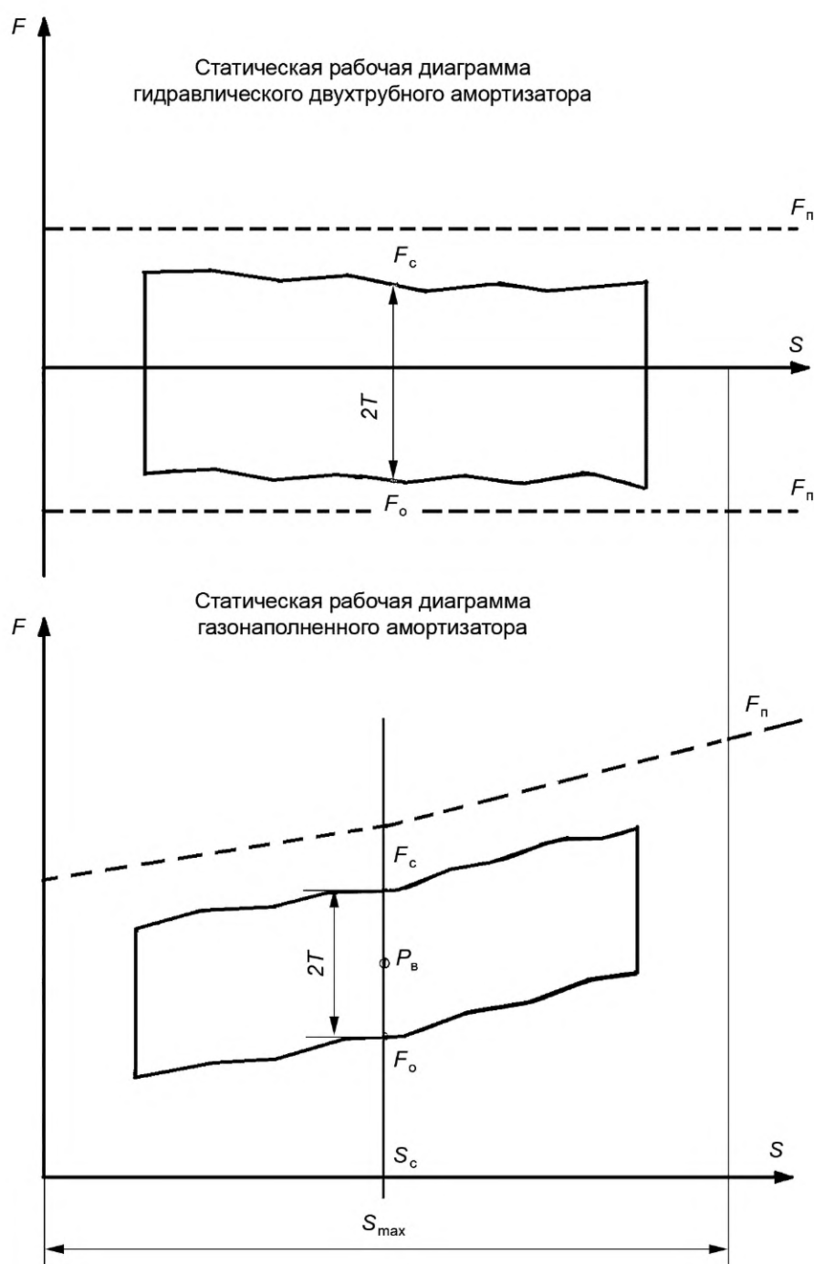
Рисунок 1 — Статические рабочие диаграммы амортизаторов
