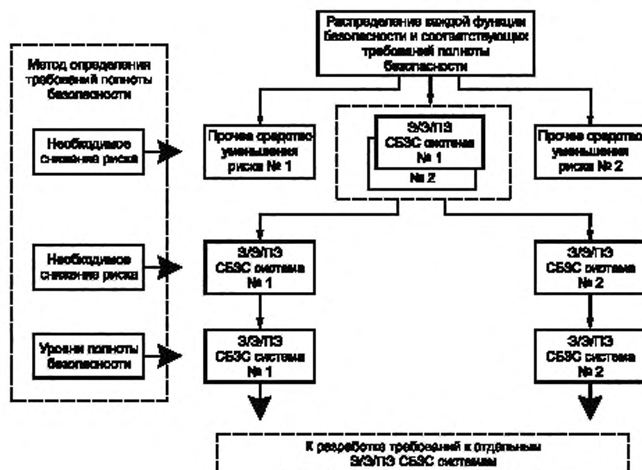
Рисунок 2 — Распределение функции безопасности по Э/Э/ПЗ СБЗС системам и прочим средствам уменьшения риска
