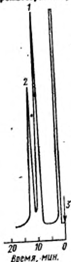
Хроматограмма фенолоформальдегидных смол
