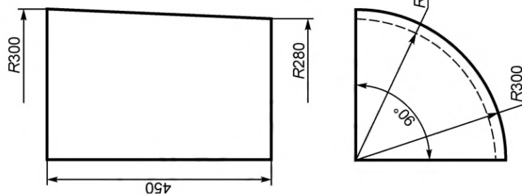
Рисунок 9 — Фасонное изделие номер 74 (для пробки купола)
