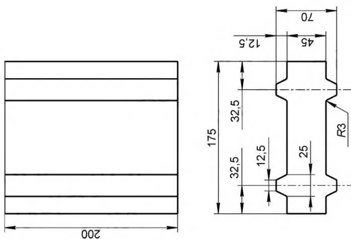
Рисунок 10 — Фасонное изделие номер 79 (насадочное)
