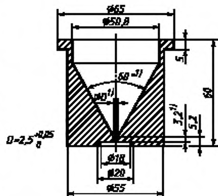
Рисунок 1 — Калиброванная воронка (прибор Холла)
