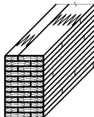
б) Однослойный деревянный клееный элемент
